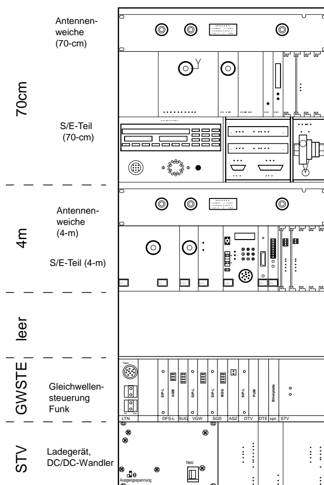
Beispiel: FSO-BOS Prinzipaufbau
